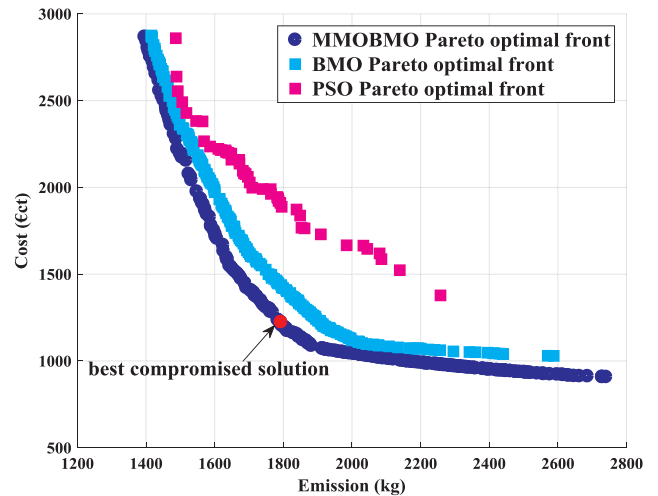
Fig. 16. Pareto optimal fronts of MMOBMO, BMO and PSO: first sub-scenario (first scenario).
