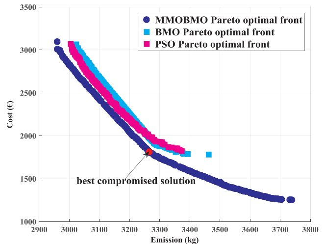
Fig. 17. Pareto optimal fronts of MMOBMO, BMO and PSO: second sub-scenario (first scenario).
