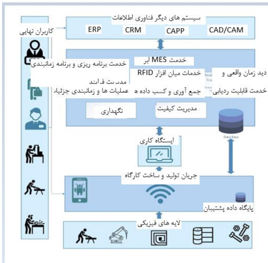
شکل 1: معماری MES هوشمند
